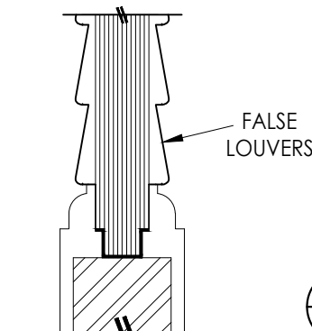
FALSE LOUVER OPTION
